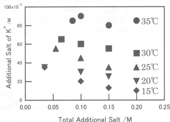
図1. \kappa カラゲナン水溶液のゾルゲル転移相図。ナトリウム塩型 \kappa カラゲナンを用い、水溶液濃度は0.5wt%。
