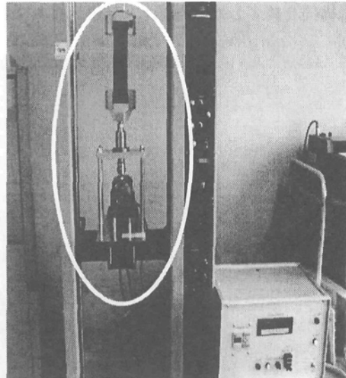
図1. 繰り返し試験機試作部分
