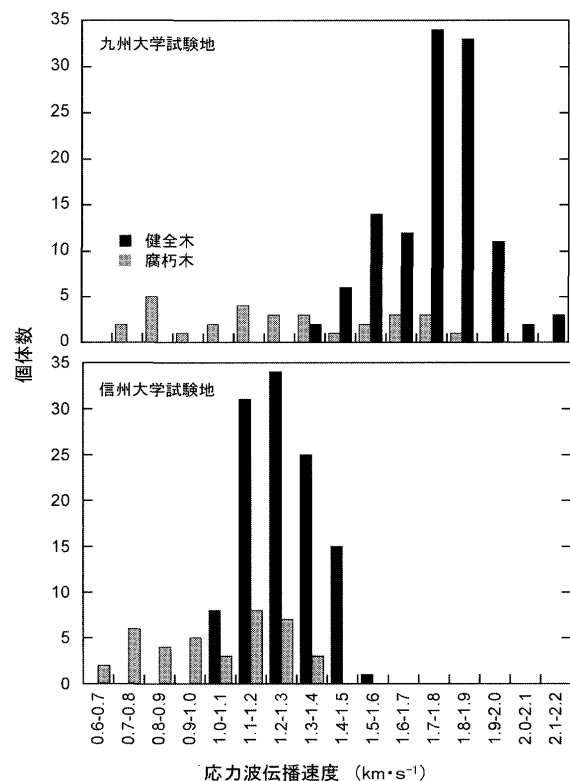
図-2. 健全木と腐朽木の応力波伝播速度のヒストグラム
