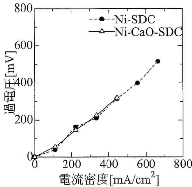
図 2. エタノール発電時の Ni-SDC と Ni-CaO-SDC 燃料極の電流-過電圧特性
