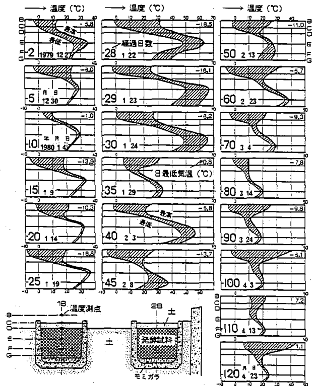
図9 中央発酵中央測線 (18) の鉛直方向温度分布 (O～O断面)
