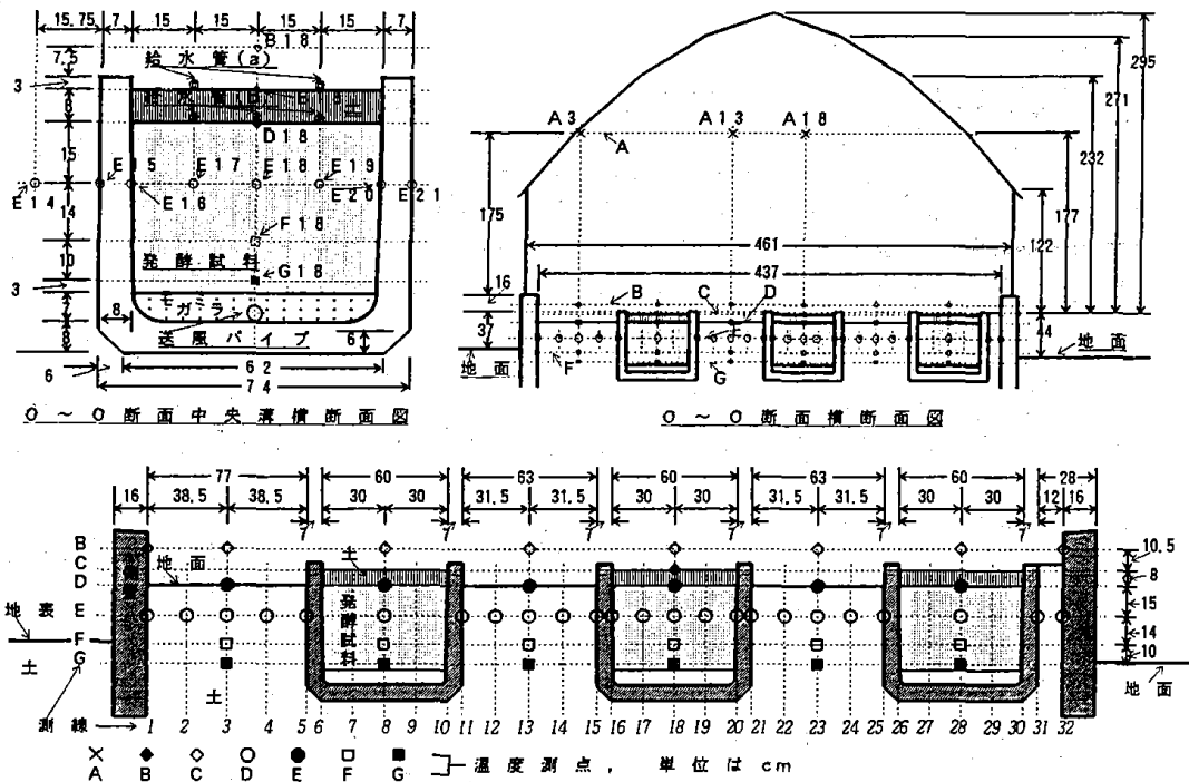
図2 [O~O断面] 断面図および温度測点
