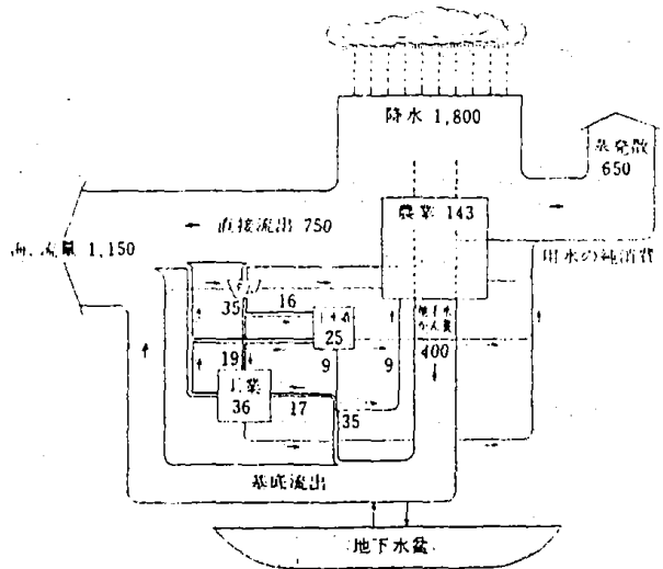
図-1 日本の水収支 (単位: mm/年) (概根 第.1977)
