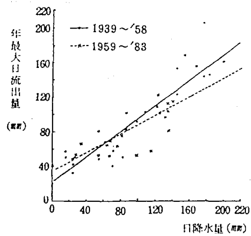
図-4 年最大日流出量と当日日降水量の関係
