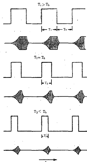
第2図 pulsetime 短縮に伴う波形の変化
