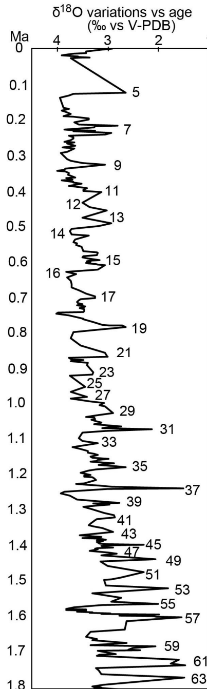
図 1 縦軸を年代とした酸素同位体比変動曲線 (U1352B 上部 500 m)
