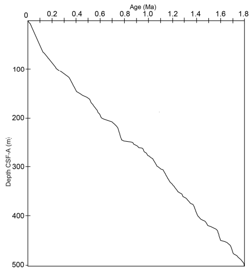
図2 U1352Bの堆積速度曲線 (年代モデル)
