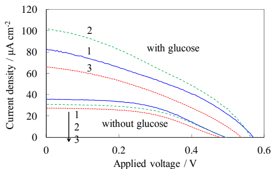
図4 (1) 酸化チタン電極、(2) 0.10%アロフェン複合電極、(3) 1.0%アロフェン複合電極を用い、グルコースを含まないまたは含む電解液中で測定した電流 - 電圧曲線
