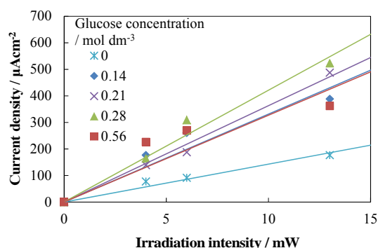
図6 0.10%アロフェン - 酸化チタン電極を用いて、各グルコース濃度の電解液中で測定した、光電流密度の光照射強度依存性
