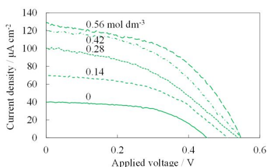
図5 0.10%アロフェン - 酸化チタン電極を用いて測定した、電流電圧曲線のでんぷん濃度依存性
