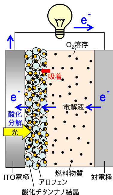
図2 本課題の光燃料電池の概念図
