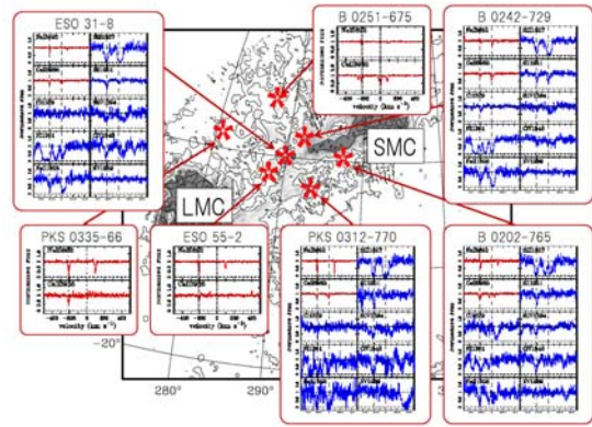
図 2 : 多視線分光観測の結果。赤が可視、青が紫外スペクトルを表す。S/N 比が低いスペクトルも含まれている。
