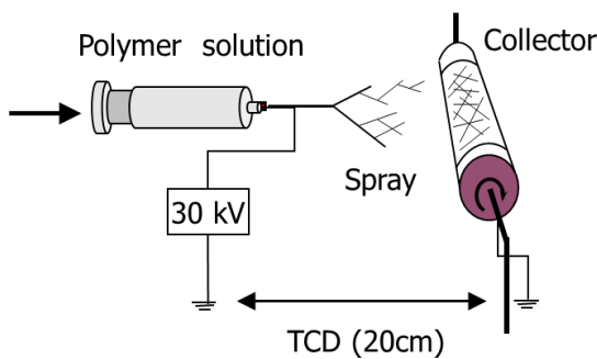
図1. NCFSの作製
