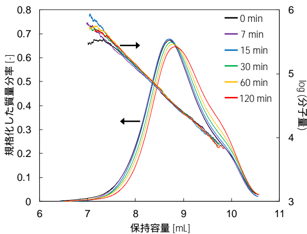
図4. セルロースナノファイバーを原料としたハイドロゲルの溶出体積と規格化した質量分率及び分子量の関係（160 処理）
