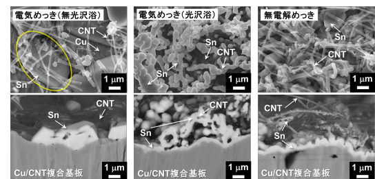
図1 Cu/CNT複合基板上にSnを析出させた負極構造体の表面・断面電子顕微鏡像。
