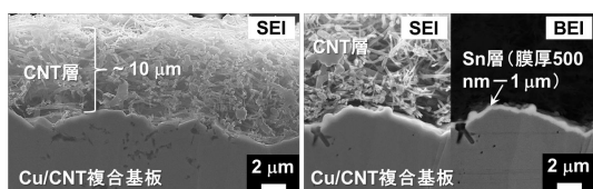
図2 複合基板上にCNTを電気泳動法により固定化した後に Sn めっき処理を施して作製した電極の断面電子顕微鏡像。(左) Sn めっき前、(右) めっき後(後方散乱電子像により Sn めっき膜の部位を特定した)
