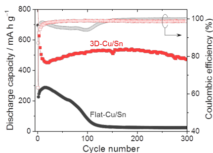
図5 三次元多孔質 Cu 上に Sn めっきした電極のサイクル性能。比較として平滑な集電体にめっきした場合のサイクル性能もあわせて示す。
