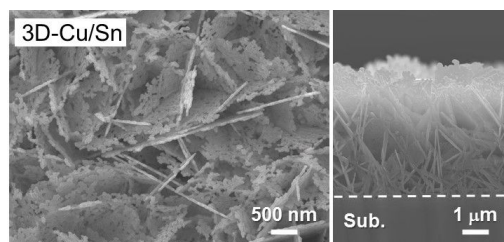
図4 PAA 添加 Cu めっき浴から作製した三次元 Cu に対して Sn めっき処理を施した電極構造体の電子顕微鏡像。
