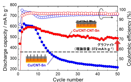
図3 電気泳動法を用いて作製した Cu/CNT-Sn 電極のサイクル性能。
