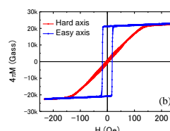
図5. FeCo 薄膜の磁化曲線。(a), FeCo 単層膜 ; (b), FeCo(100nm)/CoNi(2nm).
