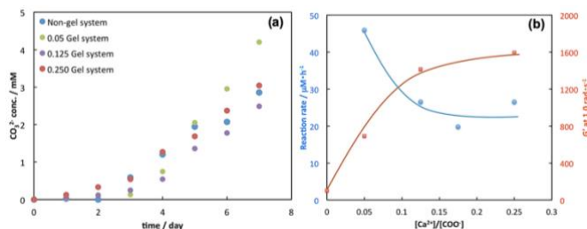
図 3 (a)各系における尿素の加水分解活性と(b)反応速度と貯蔵弾性率間での相関。
