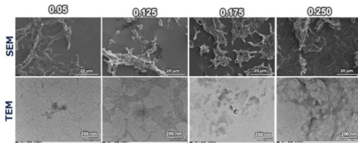
図 4 生体模倣型ミネラリゼーションにより鉱化した炭酸カルシウムのSEMおよびTEM像。
